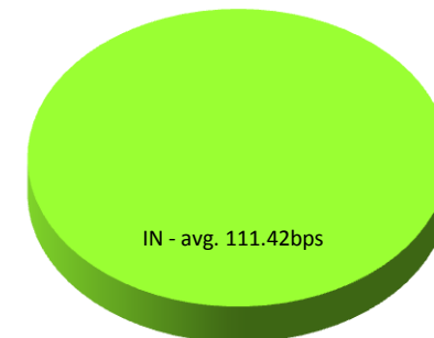
KANSUBK(8545.OS)
