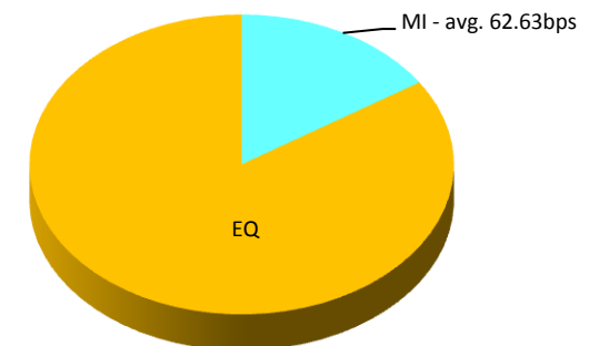
KANSUBK(8545.OS)
